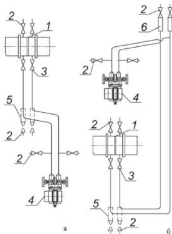
Рисунок 3.8 – Схемы соединительных линий при измерении расхода жидкости
