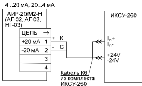
Рисунок 3.2 – Схема электрическая подключений.
