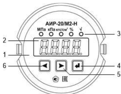
Рисунок 2.2 – Общий вид передней панели AIR-20/M2-H с СД-индикатором
