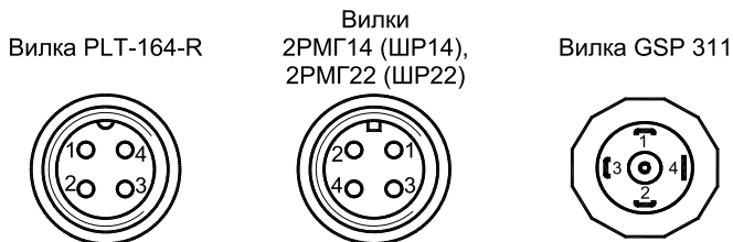
Рисунок 2.3 – Расположение контактов вилок
