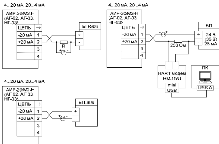
Рисунок 3.2 – Схема электрическая подключений.
