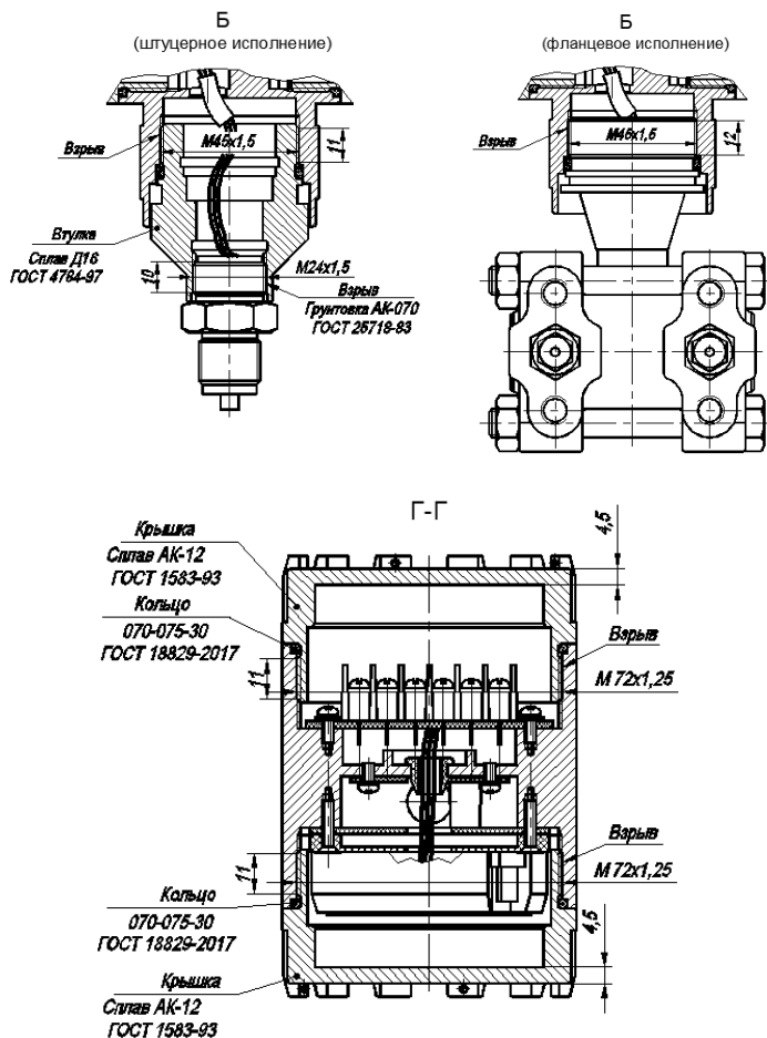
Рисунок А.4 – Чертеж средств взрывозащиты
