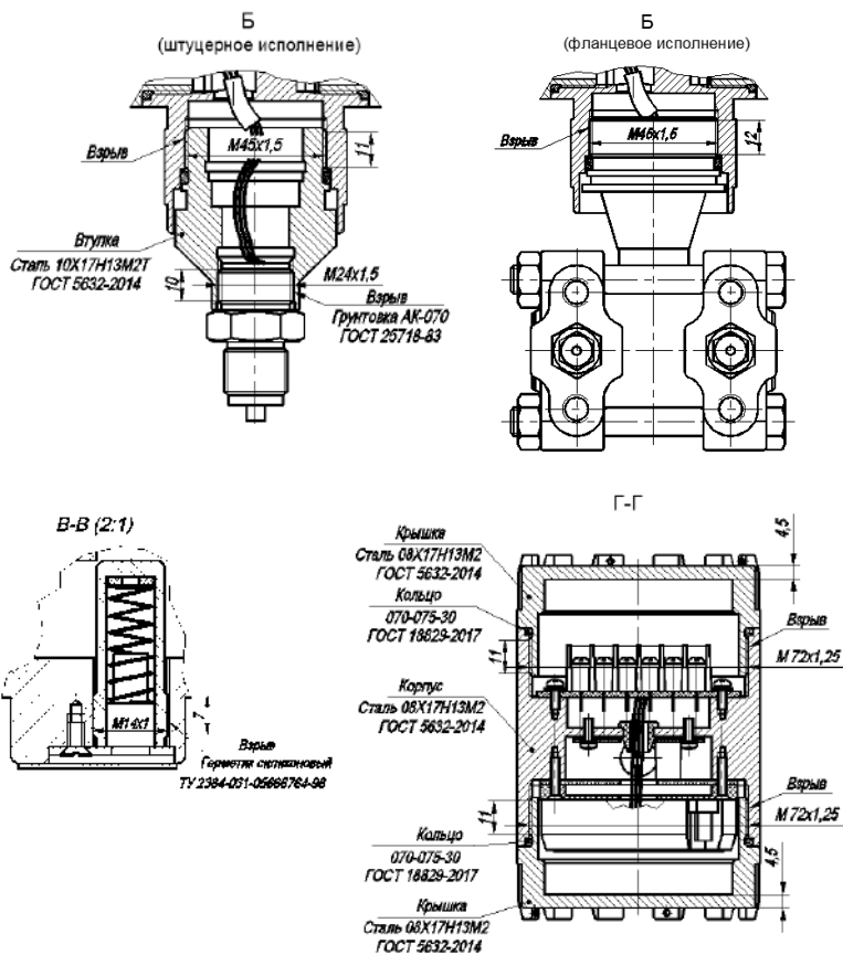
Рисунок А.7 – Чертеж средств взрывозащиты
