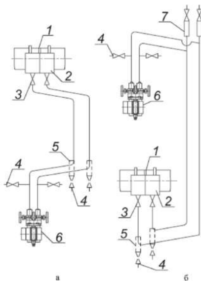
Рисунок 3.7 – Схемы импульсных линий при измерении расхода пара
